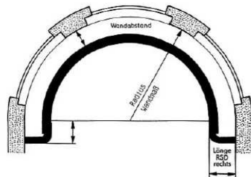
Sonderbiegung
